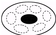
Рис. 4. Двухмерный циклический аттрактор (Торас)
