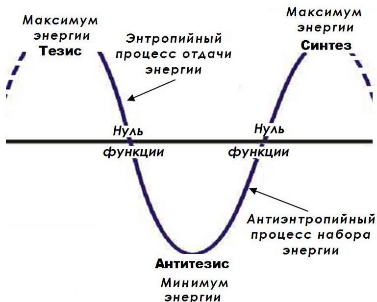
Рис. 29. Динамика взаимного перехода жизни и смерти
