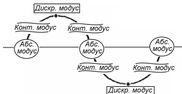
Рис. 1. Три модуса бытия, отраженные в структуре волны
