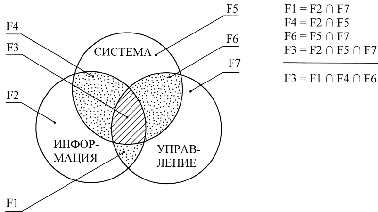
Рис. В.2. Логическая триада процесса мышления: F1 — поле информационно-управляющее; F2 — поле информационное; F3 — поле «сигма»; F4 — поле информационно-системное; F5 — поле системное; F6 — поле системно-управляющее; F7 — поле управляющее
