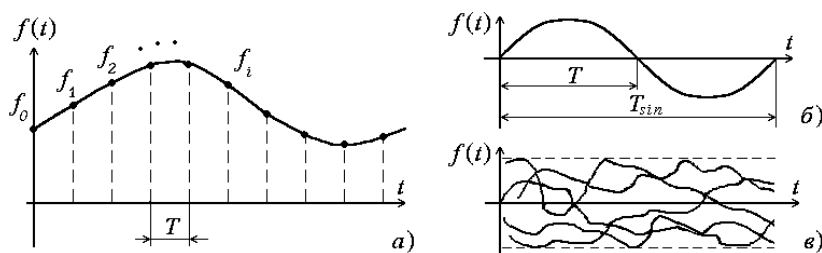
Рис. 2.9. Иллюстрация к теореме Котельникова
