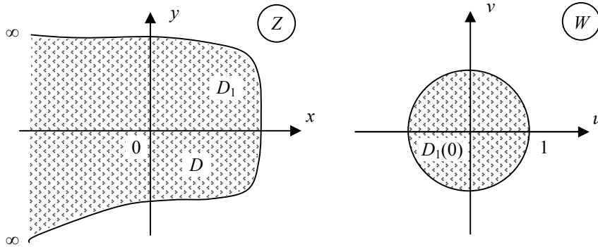
Рис. 2.20. К иллюстрации теоремы 2.9 ( D_1 — произвольно заданная в D точка)
