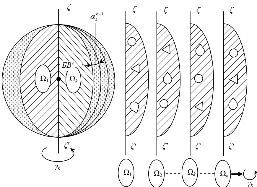
Рис. 2.28. Иллюстрация перехода от двумерного к трехмерному компактному многообразию без краев в гипотезе Пуанкаре
