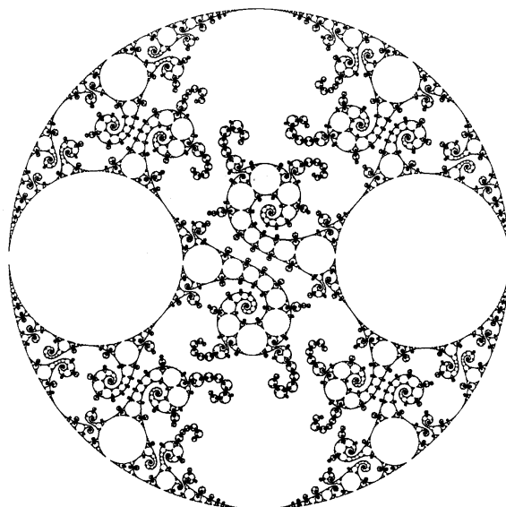
Рис. 3.5. К иллюстрации плотности вернадскиана: из книги Б. Мандельброта 172 — самогомографический фрактал (вблизи предела Пеано); гомография, или гомография Мёбиуса (см. § 2.4), отображает плотность по закону дробно-линейного преобразования
