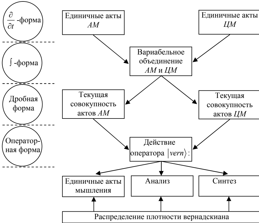
Рис. 3.4. Схема описания процессов в функциональном пространстве M(\tau) с учетом плотности оператора вернадскиана
