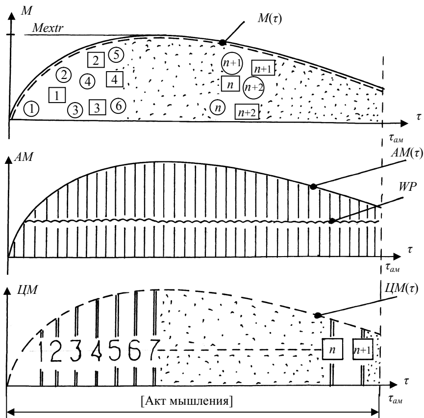
Рис. 2.15. Двумерная геометризация единичного акта мышления: на эпюре M(\tau) — суммарный акт; на эпюрах AM(\tau) и ЦМ(\tau) — акты аналогового и цифрового мышления, соответственно; \textcircled{i} и \boxed{i} — единичные группы CT_i ЭМВ в процессах аналогового и цифрового мышления, соответственно; WP (wave process) — условное графическое обозначение того, что AM(\tau) является волновым (солитонным) непрерывным процессом; заштрихованные области на эпюрах M(\tau) и ЦМ(\tau) обозначают продолжение и окончание процессов акта мышления; 1, 2, 3, ..., n , n+1 , ... — на эпюре ЦМ(\tau) обозначают единичные CT_i ЭМВ, или их паттерны; \tau_{ам} — длительность акта мышления; M_{extr} — (локальный) экстремум в единичном акте мышления
