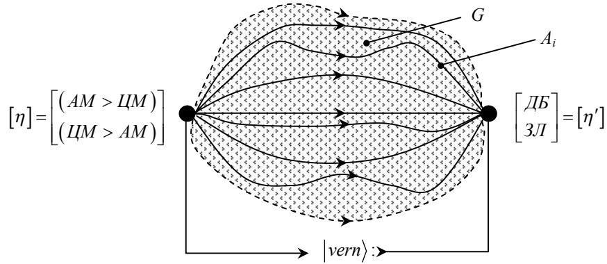
Рис. 3.1. К иллюстрации теоремы 3.1: амплитуды перехода от матрицы-столбца \eta к матрице-столбцу \eta' ; G — область действия процесса
