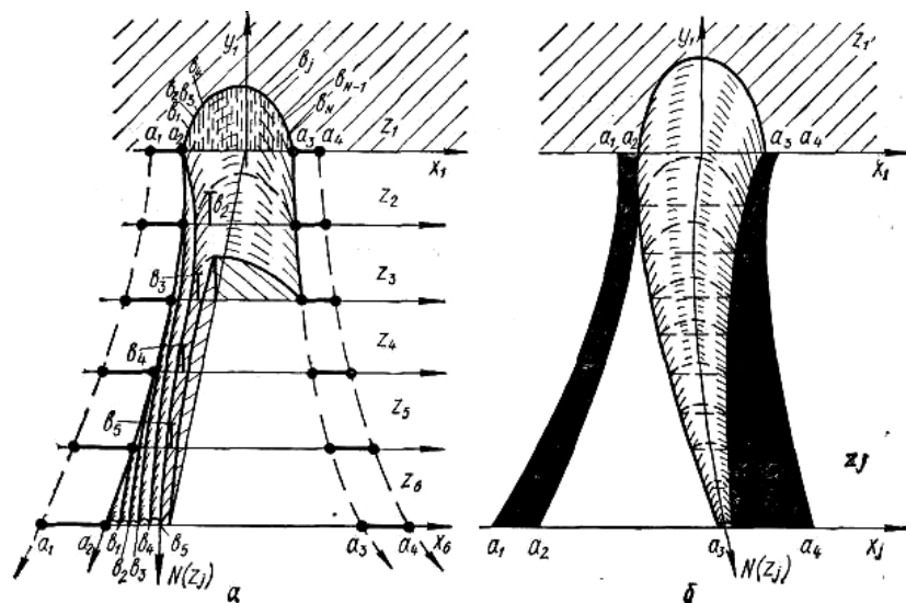
Рис. 2.25. Графическое изображение алгоритма ПКО последовательных Re -стягиваний
