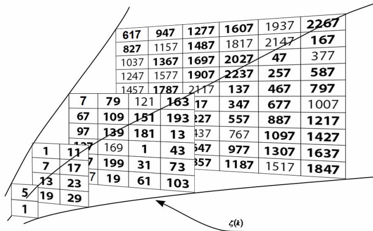
Рис. В.3. Несколько первых «разреженных» матриц простых чисел, полученных по алгоритму (B. 22), (B.23) ( \zeta(k) — функция расширения матриц); простые числа выделены жирным
