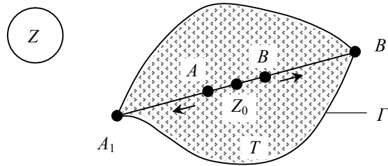
Рис. 2.19. К доказательству теоремы 2.8
