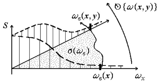
Рис. 2.12. К изменению спектра S(\omega) в реальной среде распространения сигнала
