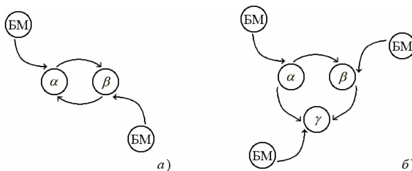
Рис. 2.8. Примеры гиперциклов Эйгена-Шустера: возникновение биомолекул \alpha , \beta в результате автокаталитической реакции из биоматериала (БМ) (а); цикл с участием трех типов биомолекул \alpha , \beta , \gamma (б)
