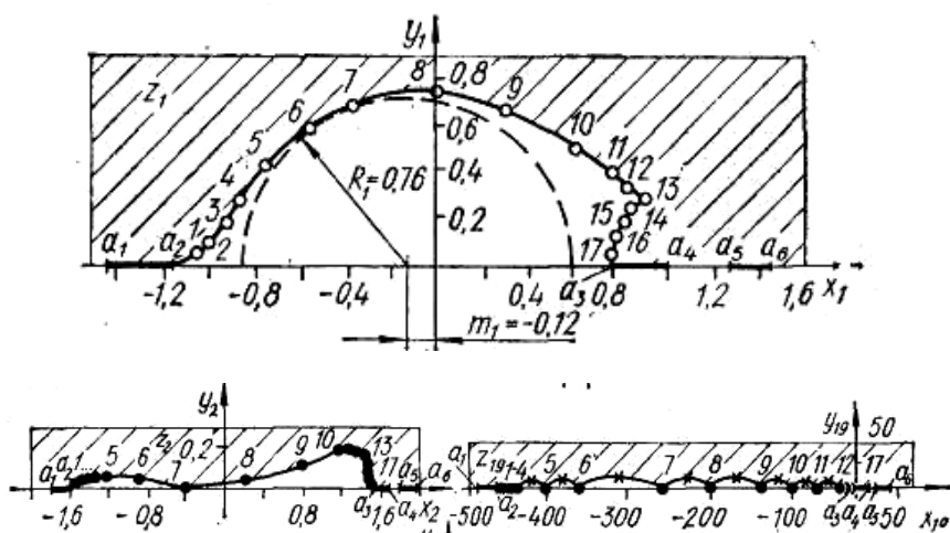
Рис. 2.24. К иллюстрации алгоритма ПКО последовательных Re -стягиваний
