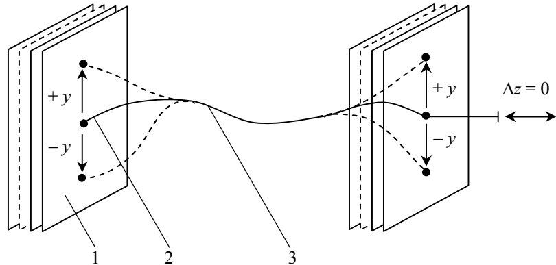
Рис. 3.9. Иллюстрация к понятию Д-браны: 1 — Д-брана (гиперповерхность); 2 — свободный конец открытой струны 3. Вдоль Д-браны концы струны свободно перемещаются \pm y , однако в поперечном z -направлении свободного перемещения нет ( \Delta z = 0 ).
