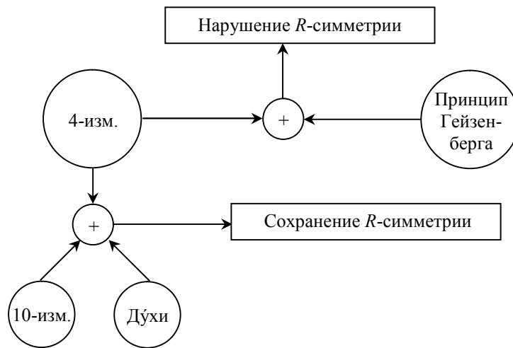
Рис. 3.6. Диаграмма, поясняющая принцип сохранения R -симметрии
