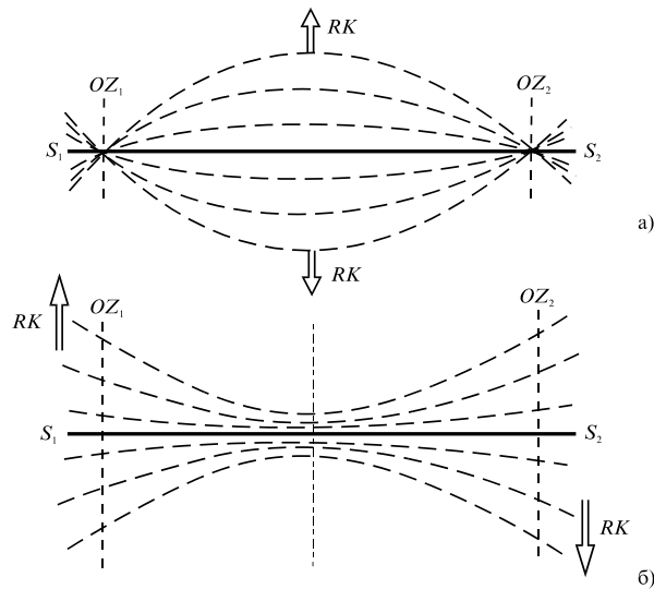
Рис. 3.13. К генерации мировых листов закрепленной (а) и незакрепленной (б) суперструнами
