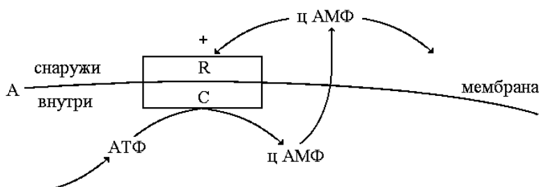
Рис. 2.4. Механизм колебательного синтеза цАМФ у амёбы Dictyostelium discoideum
