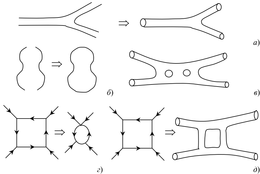
Рис. 3.7. Диаграммы, поясняющие сущность действия струн: вершины взаимодействия открытых струн, переходящие ( \Rightarrow ) в вершины замкнутых струн (а); появление замкнутых струн в результате взаимодействия двух открытых струн (б); двухпетлевая диаграмма Фейнмана для рассеяния замкнутых струн (без учета ультрафиолетовой расходимости*) (в); однопетлевая диаграмма Фейнмана для четырехчастичного рассеяния (ультрафиолетовая расходимость здесь соответствует стягиванию в точку одной внутренней линии) (г); изменение диаграммы (Фейнмана) при переходе от квантовой гравитации к теории струн (суперструн) (д)
