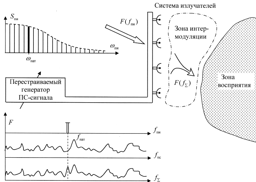
Рис. 1.5. Модельная схема, поясняющая лемму 1.4, использующая радиофизические аналогии
