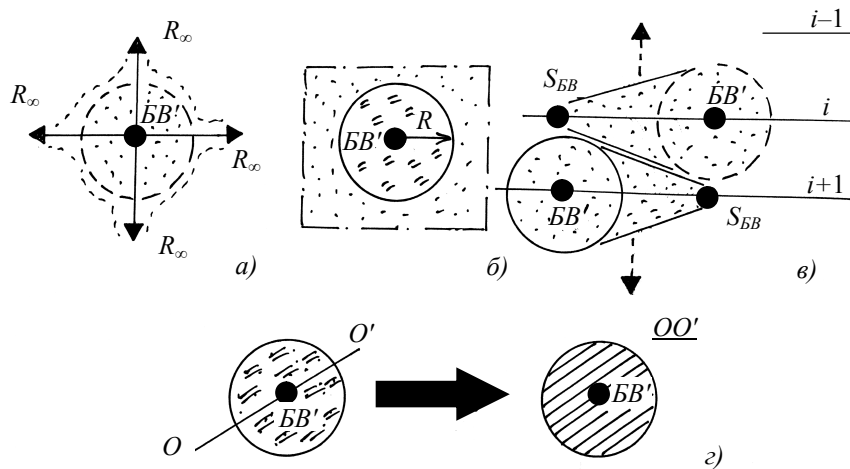
Рис. 2.22. К иллюстрации гипотезы Пуанкаре в существующих концепциях геометрофизики Вселенной: бесконечная (бесконечно расширяющаяся) Вселенная (а); конечная Вселенная в «пустоте» (б); концепция пульсирующих Вселенных (в); диаметрально сечение OO' конечной Вселенной (г); BB' — «точка» бывшего Большого взрыва 83 ; S_{BB} — сингулярность (горячего) Большого взрыва; i — номера пульсирующих (множественных) вселенных; заштрихованы: точками — изменяющиеся размеры (объемы) Вселенной в концепциях (а), (б) и (в); двойными штрихами — объемы конечной Вселенной в (б) и (г); сплошными линиями — диаметрально сечение OO' конечной Вселенной
