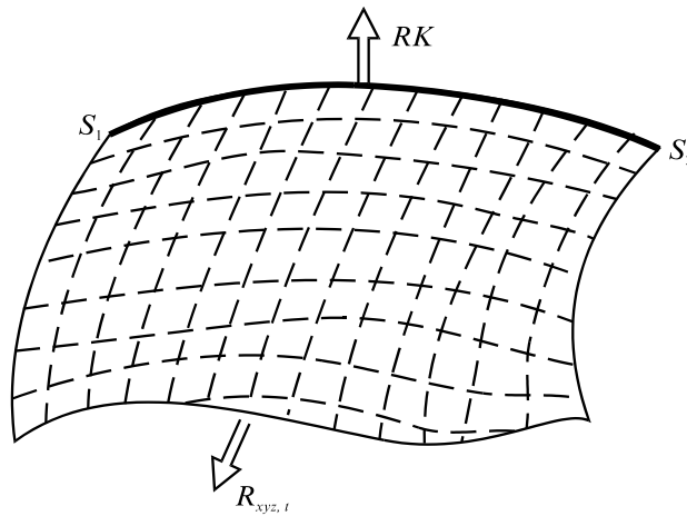
Рис. 3.14. Генерируемый суперструной мировой лист
