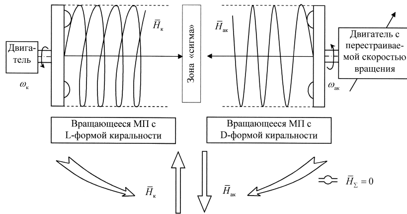
Рис. В. 1. Схема биофизического эксперимента, иллюстрирующего на примере пространственного взаимодействия киральных магнитных полей (МП) совместную работу правого и левого полушарий головного мозга человека
