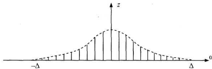
Рис. 2.14. К выводу теоремы Котельникова
