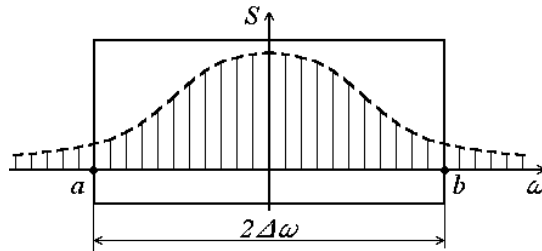
Рис. 2.10. К иллюстрации окна наблюдения для спектра нешумовой функции
