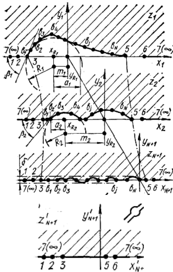
Рис. 2.26. Алгоритм ПКQ квазиканонизации R_{\text{ин}}\text{-} кругом
