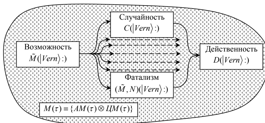
Рис. 3.2. К иллюстрации действия оператора вейнбаха в функциональном пространстве двойственности мышления с распределением возможности и ее сходимости к действительности (заштрихована зона функционального пространства)
