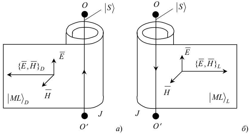
Рис. 3.10. Физические зарядовые струны и порождаемые ими ЭМП с правым вращением мирового листа |ML\rangle_D (а) и с левым |ML\rangle_L (б)
