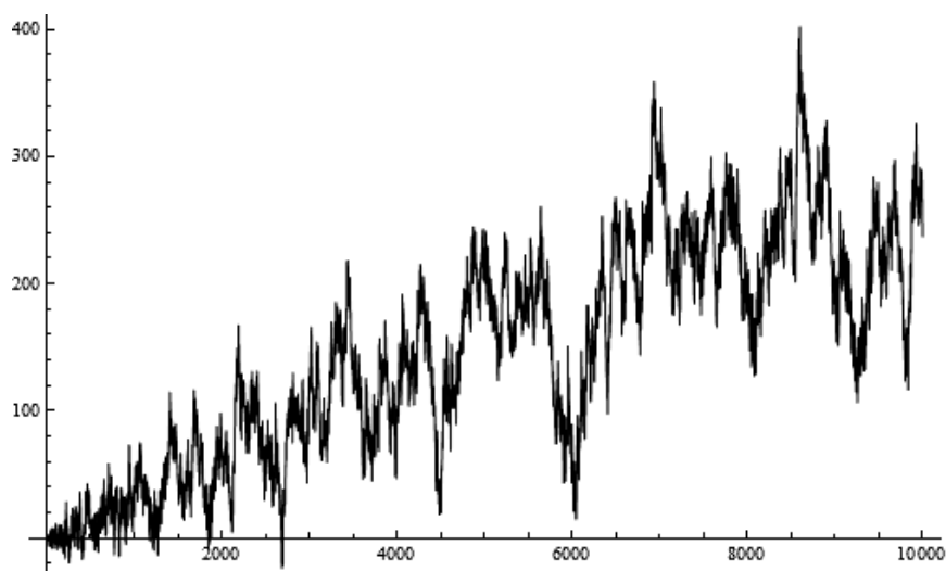
Рис. В.5. Разность между реальными и приближенными значениями для первых 10000 простых чисел. По оси абсцисс отложены номера (не напоминает ли этот график энцефалограмму?)
