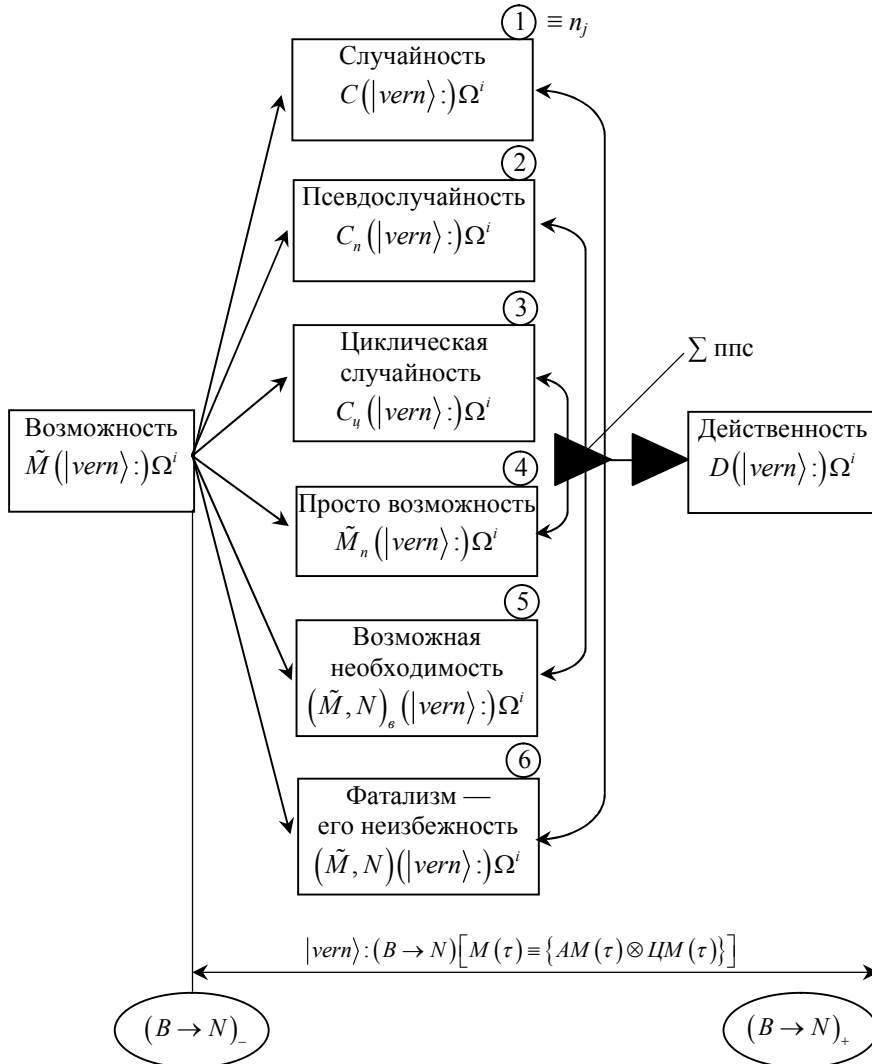
Рис. 3.3. К иллюстрации примера действия теоремы 3.3 (в конкретизацию схемы на рис. 3.2)
