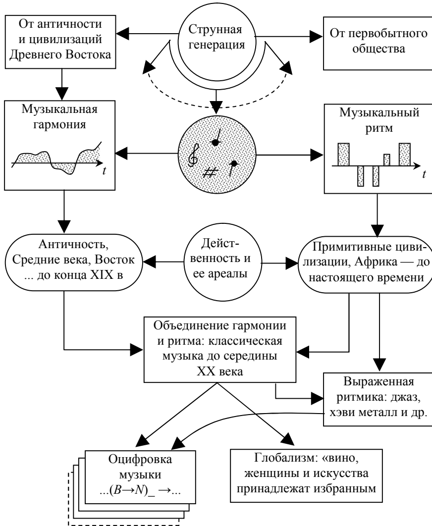
Рис. 3.16. Струнная генерация в оцифровывании музыки и связь между гармонией и ритмом
