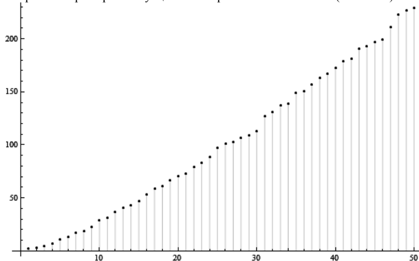
Рис. В. 4. Соответствие между номером простого числа и его значением. По оси абсцисс отложен номер простых чисел, по оси ординат — значения простых чисел.
