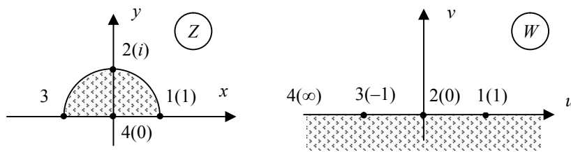
Рис. 2.21. Взаимнооднозначное отображение полуплоскости на полукруг
