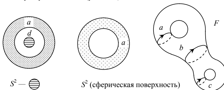
Рис. 2.18. К иллюстрации понятия фундаментальной группы Пуанкаре (по Мацуо Комацу 176 )
