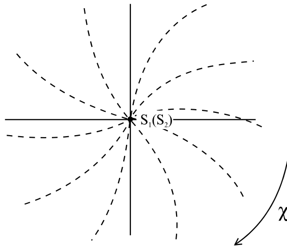
Рис. 3.15. Вращение генерируемых суперструной мировых листов
