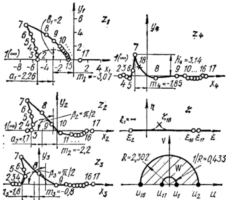
Рис. 2.27. Квазиканонизация полуплоскости с вырезанной сингулярностью с итоговым КО на полукольцо (численный пример — в относительных единицах)
