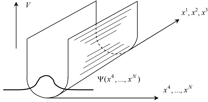
Рис. 3.11. К иллюстрации локализации волновых функций частиц на бране (по В. А. Рубакову)
