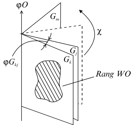
Рис. 3.12. Иллюстрация, поясняющая лемму 3.8
