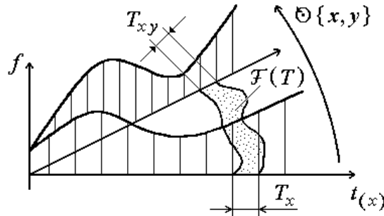
Рис. 2.13. К изменению функции f(t) в реальной среде распространения сигнала
