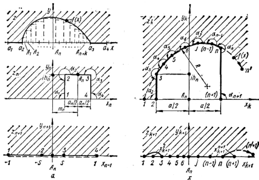
Рис. 2.23. Общая схема ПКО полуплоскости в Z с вырезанной сингулярностью (под кривой f(x) ) на полную полуплоскость с помощью AP_n -алгоритма (а) и с помощью AM_n -алгоритма (б)
