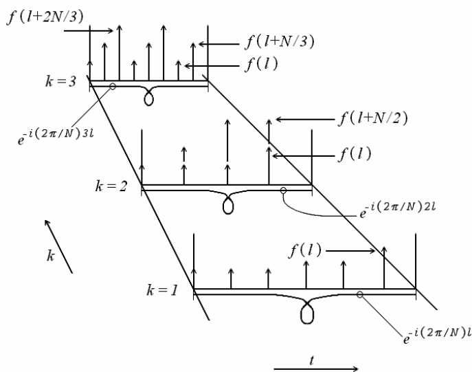
Рис. 2.11. К иллюстрации дискретного преобразования Фурье в интерпретации К. С. Overman и D.F. Mix.
