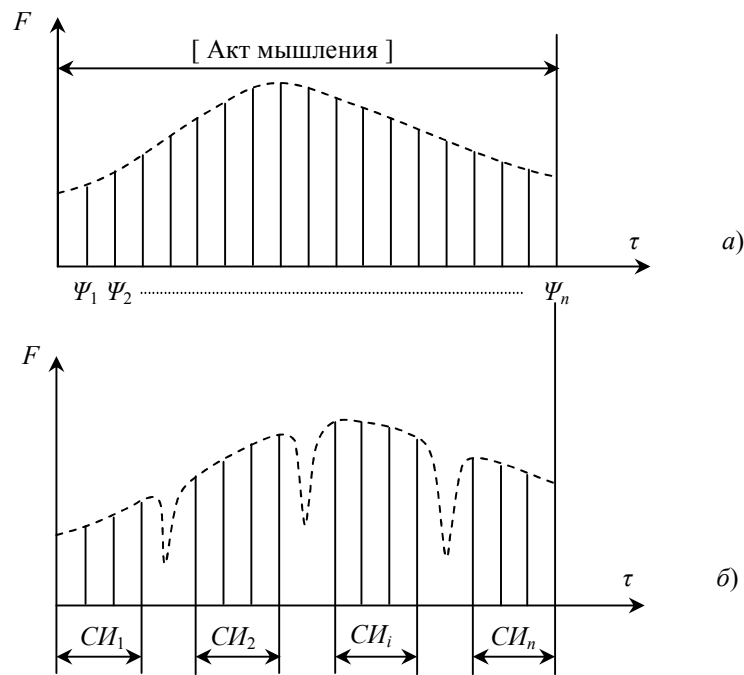
Рис. 3.17. Иллюстрация к теореме 3.5: единичный акт АМ (а) и ЦМ (б)
