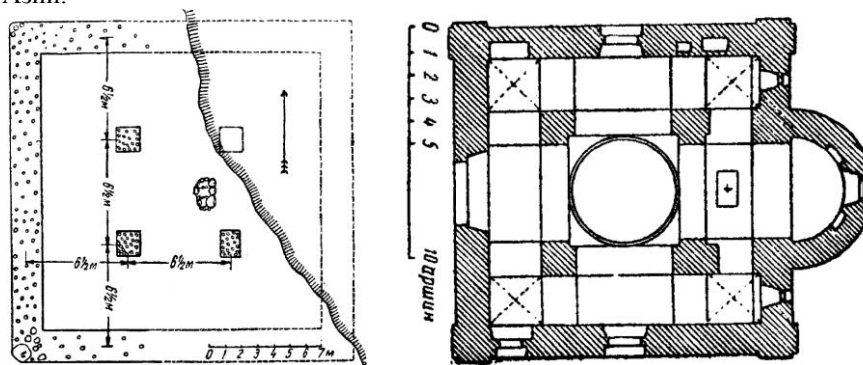
Рис. 32. Славянские храмы с четырьмя колоннами. Слева храм бога Святовита в Арконе (о. Рюген) (по [Брунов, 1944]). В храме находятся четыре столба, между которыми стоял идол Святовита, сдвинутый от центра к востоку. Справа ц. Николы на Липне в Новгороде (1292 г.) (по [Брунов, 1944]).
