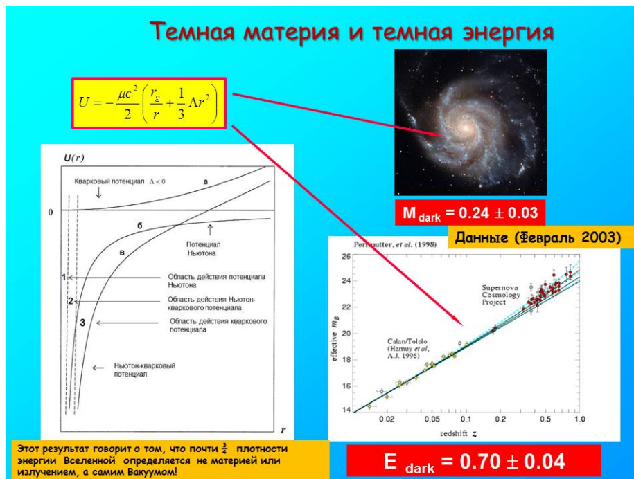
Рис. 12. Темная материя M_{dark} и темная энергия E_{dark} составляют 94% всего вещества Вселенной
