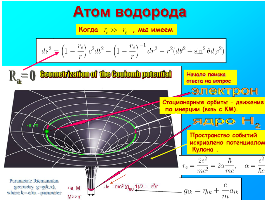
Рис.6. Стационарные орбиты в атоме водорода как геодезические искривленного риманова пространства
